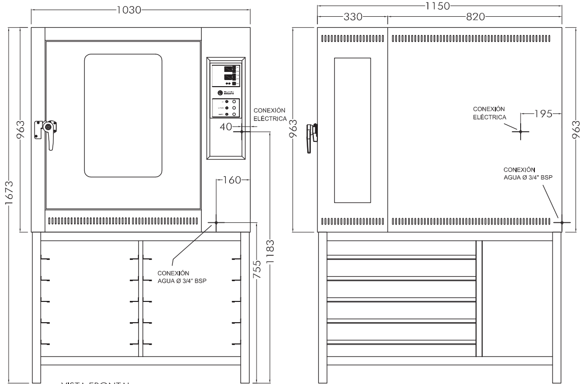
VISTA LATERAL ESC. 1:16
